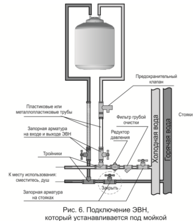
Рис. 6. Подключение ЭВН, который устанавливается под мойкой
