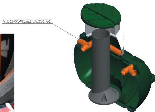
рисунок 3 Технологическое отверстие в системе орошения для вывода напорного шланга и силового кабеля
